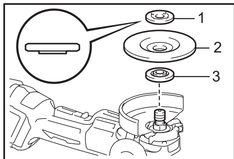
► 1. Contratuercas 2. Disco de centro hundido 3. Breda interior
