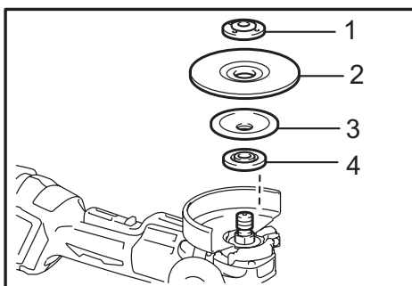
► 1. Contratuercas 2. Disco flexible 3. Plato de goma 4. Breda interior
