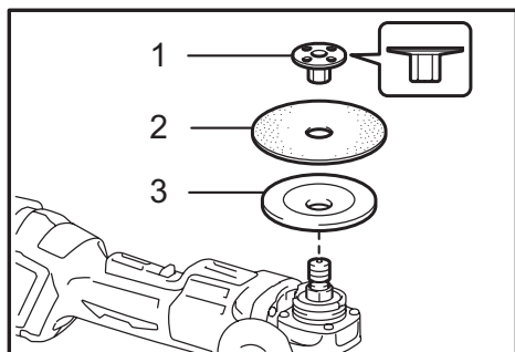
► 1. Contratuerca de lijado 2. Disco de lija 3. Plato de goma de goma
